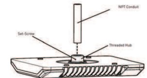
Pendant mount Installation
